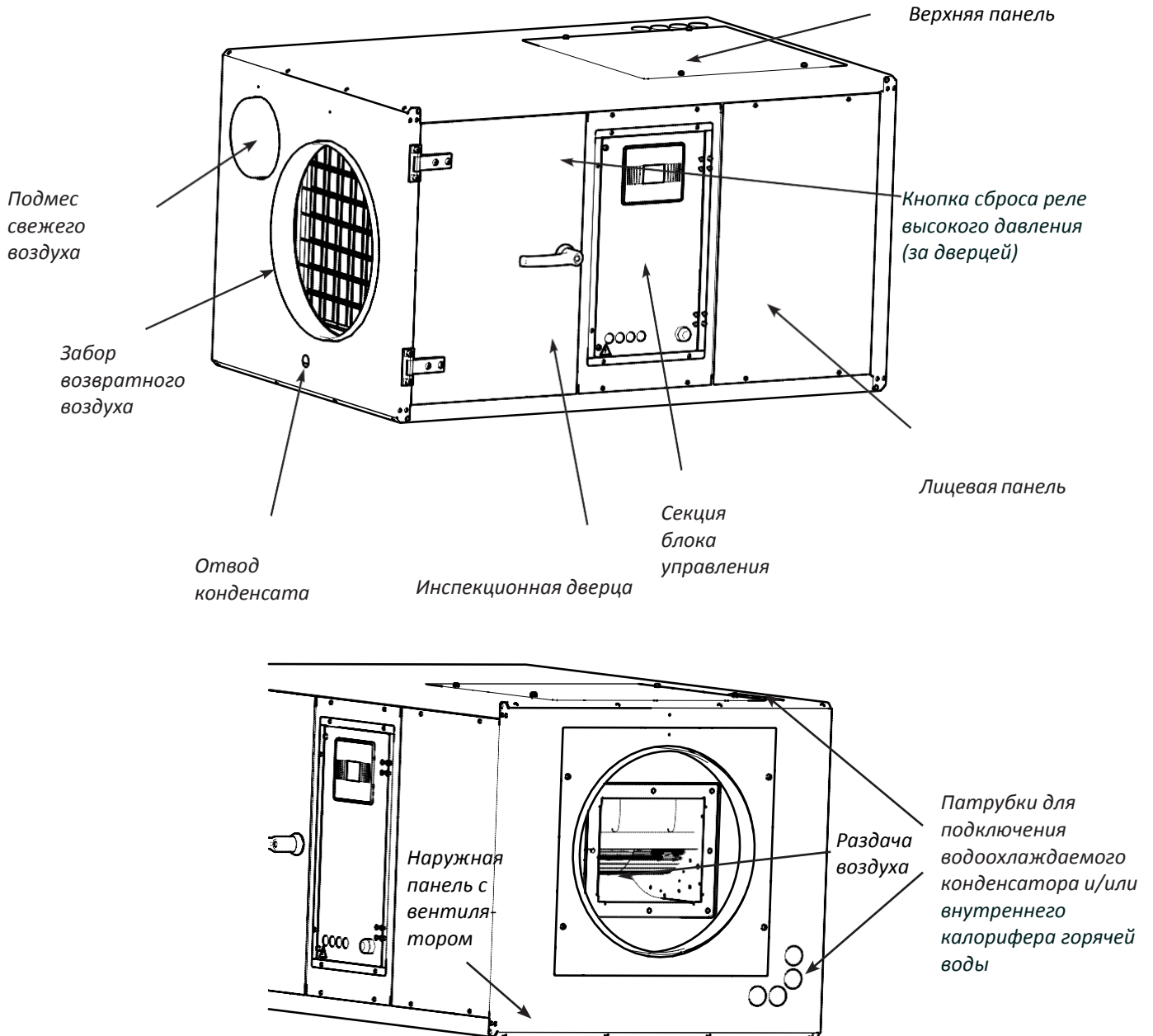
Рис. 1: Осушитель CDP
