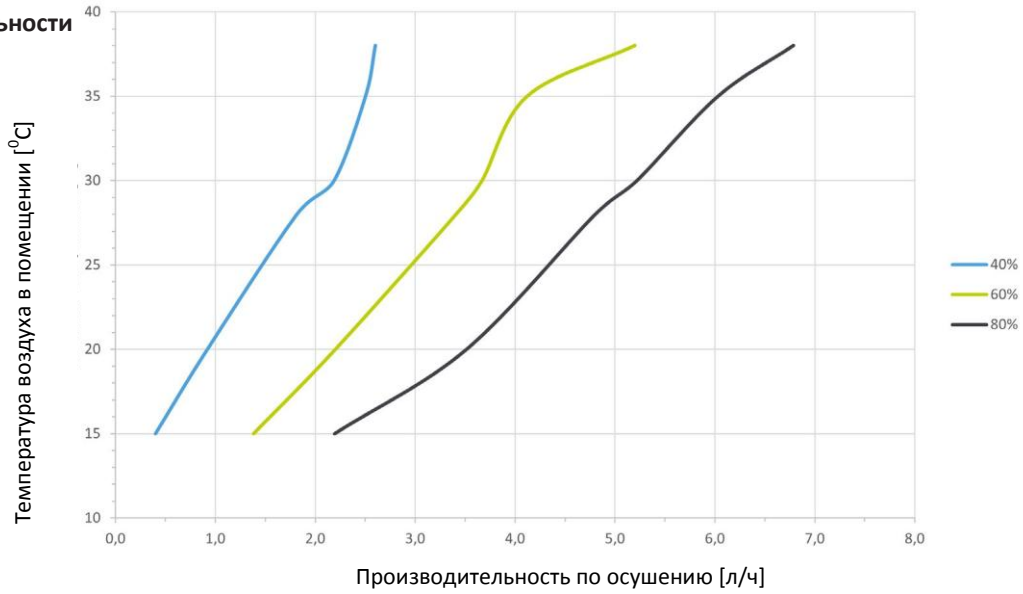
Диаграмма производительности для CDP 135 2500 м 3 /ч
